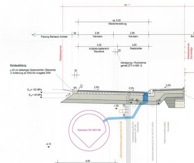
Ausbauquerschnitt Konrad-Zuse-Straße Fahrtrichtung Wiesbaden Nordenstadt Bereich Bushaltestelle
